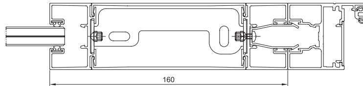
Przekrój poziomy przez słupek i ościeżnicę drzwi
